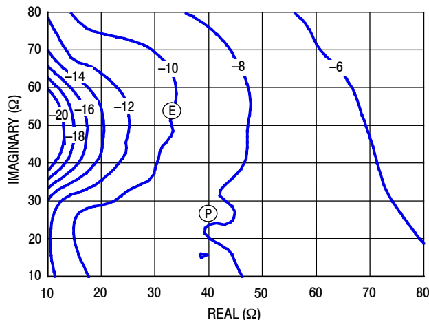
Figure 24. P1dB Load Pull AM/PM Contours (°)
